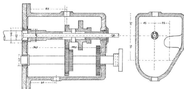
Girkassen ble tegnet med stengunløpet lagt inn som mellomaksel.
