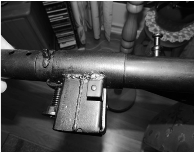
Norskprodusert Stengun med løp fra Westad.
