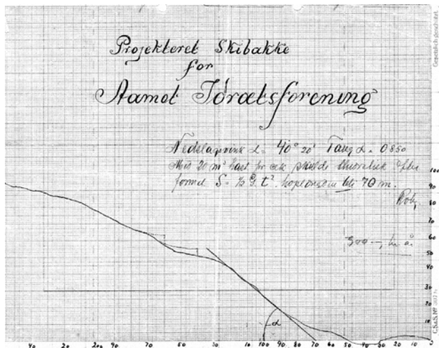
Profil av bakken som planlagt. Hopplengden ble beregnet til 70 m med nedslagsvinkel 40 grader.
