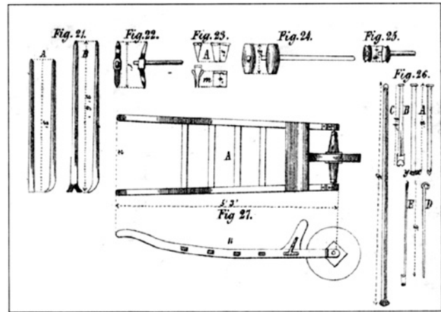
Redskaper benyttet for bryting av kalkstein. Ovenfra fra venstre er vist: Diverse brekkstenger, hakke, jernkiler, steinslegge, steinhammer, jernladestokker og minebor samt steintrillebør.
