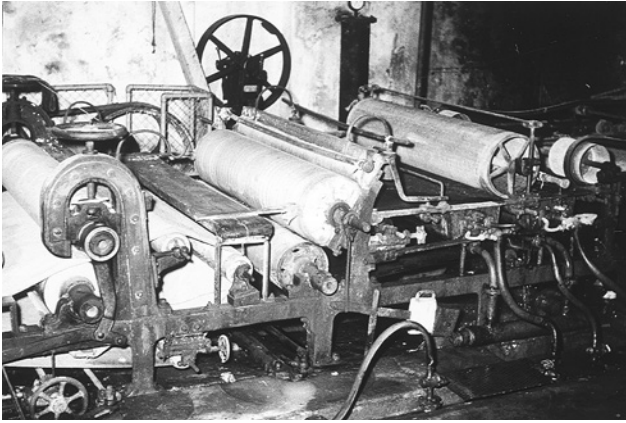
Papirmaskinen «Saksa».
