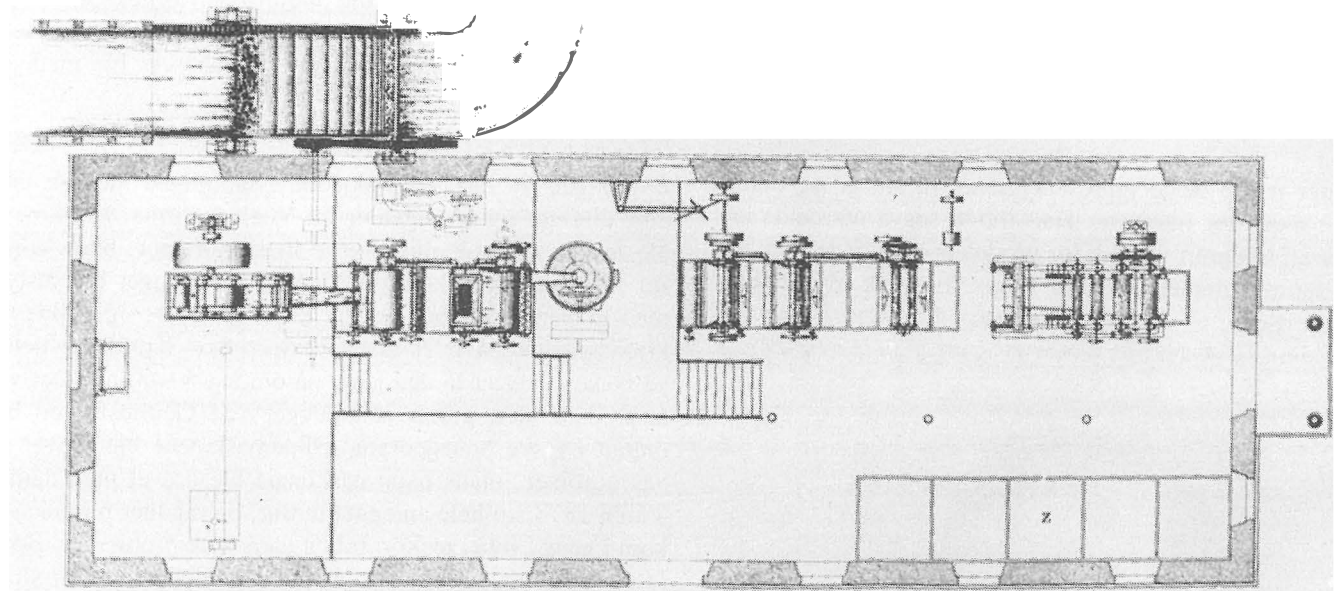
Voelters første tresliperiapparat fra 1848.
