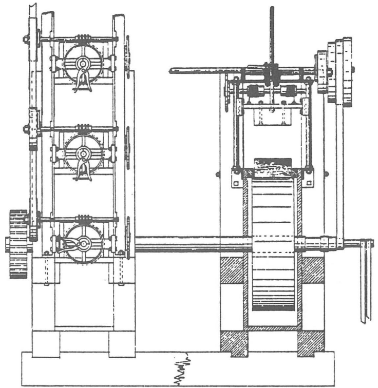
Tegning av tresliperi etter Voelters system, lik anlegget som Drammenselven bestilte i 1873.
