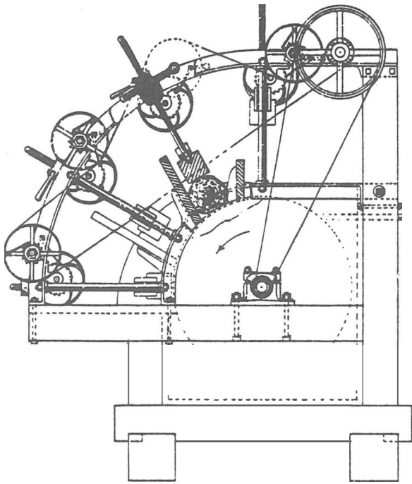
Tegning av tresliperi etter Voelters system, lik anlegget som Drammenselven bestilte i 1873.
